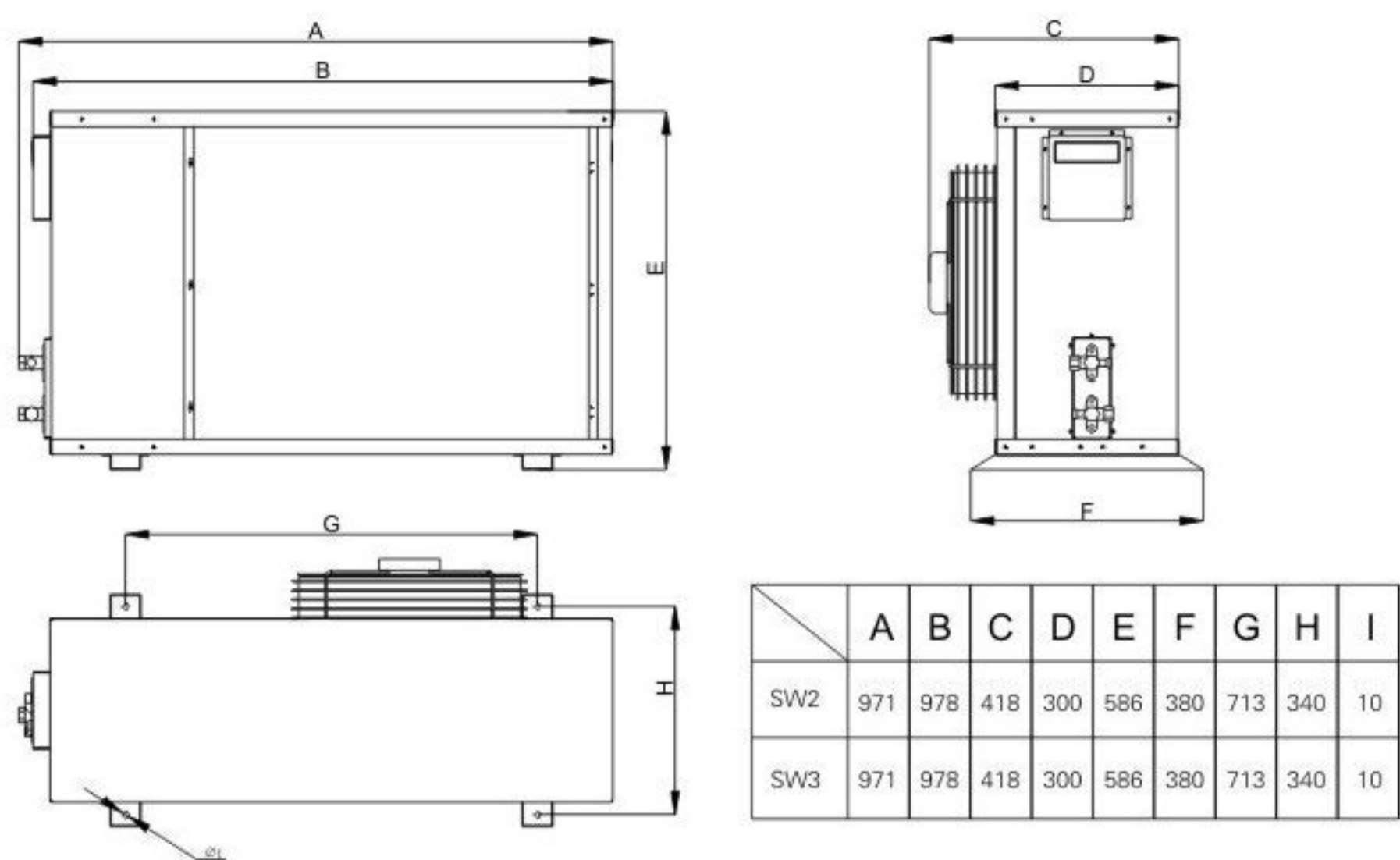
室外机
